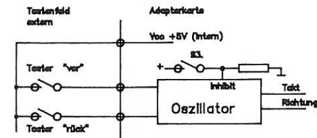
Bild 7: Beschaltung der internen Oszillatoren
