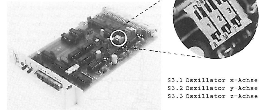
Bild 8: Platinenauszug der Oszillator-DIP-Schalter
