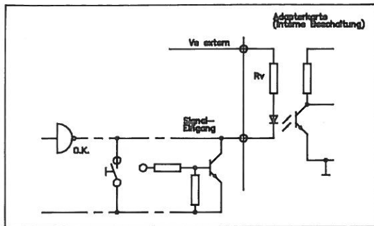
Bild 6: Ansteuerung der Opto-Koppler-Eingänge
