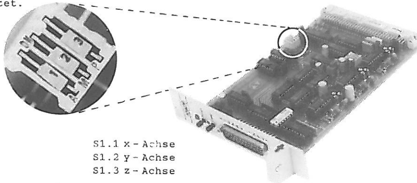
Bild 13: Zuordnung der Referenz-Taster
